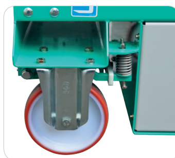
Ruote con freno automatico.
