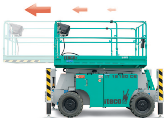
Estensione manuale piattaforma 1,4 m
