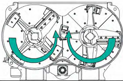
Rotazione degli assi di mescolazione sincronizzata e contrapposta
