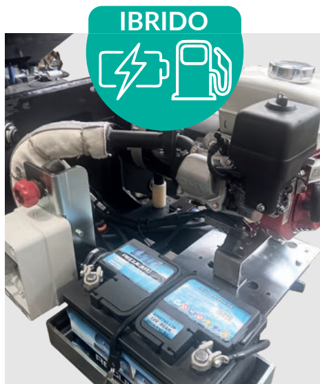
Gruppo generatore benzina e batterie litio (allestimento ibrido).
