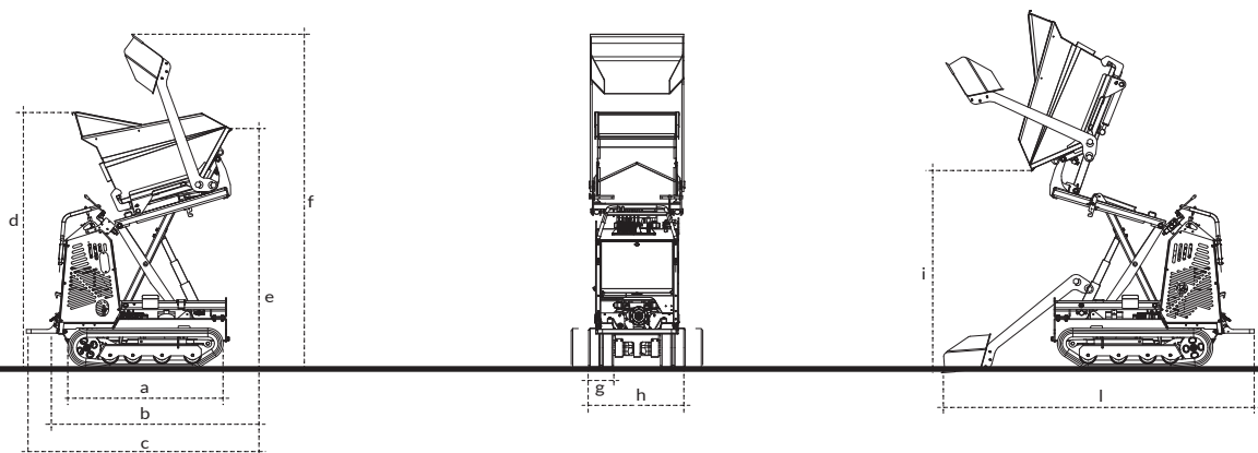
ABMESSUNGEN (mm)
