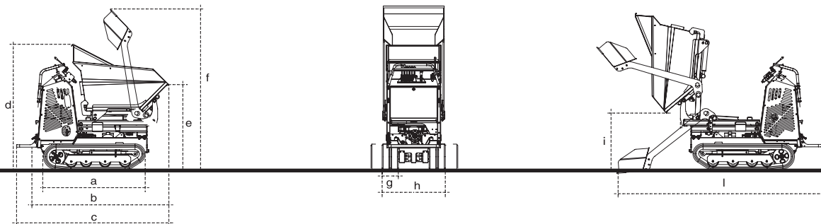
ABMESSUNGEN (mm)
