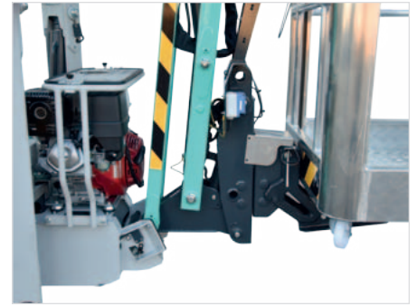
Kompaktheit der Auslegerbaugruppe, in der sich Wägezelle und das Schnellmontagesystem für Korb befindet.
